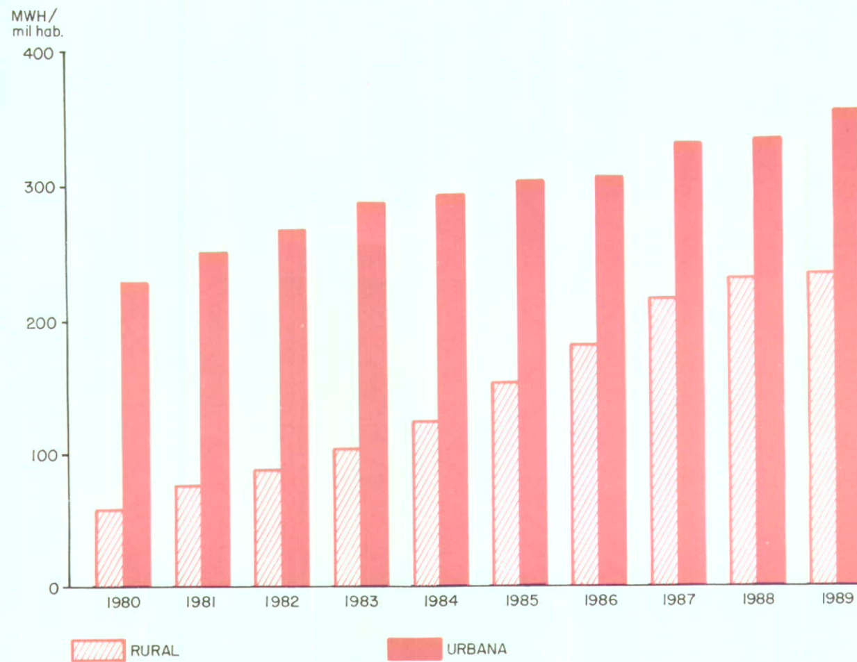
GRÁFICO 19 - CONSUMO DE ENERGIA ELÉTRICA RESIDENCIAL PER CAPITA, NAS ZONAS RURAL E URBANA, NO PARANÁ - 1980-89
