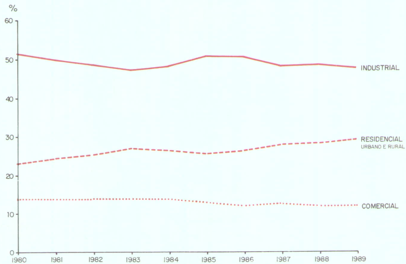
GRÁFICO 22 - PARTICIPAÇÃO DOS SETORES RESIDENCIAL, INDUSTRIAL E COMERCIAL NO CONSUMO DE ENERGIA ELÉTRICA, NO PARANÁ - 1980-89
