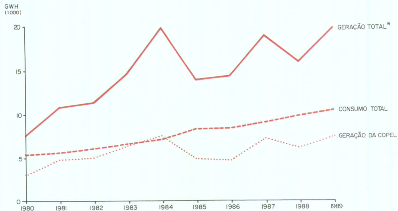
GRÁFICO 20 - GERAÇÃO E CONSUMO DE ENERGIA ELÉTRICA, NO PARANÁ - 1980-89
