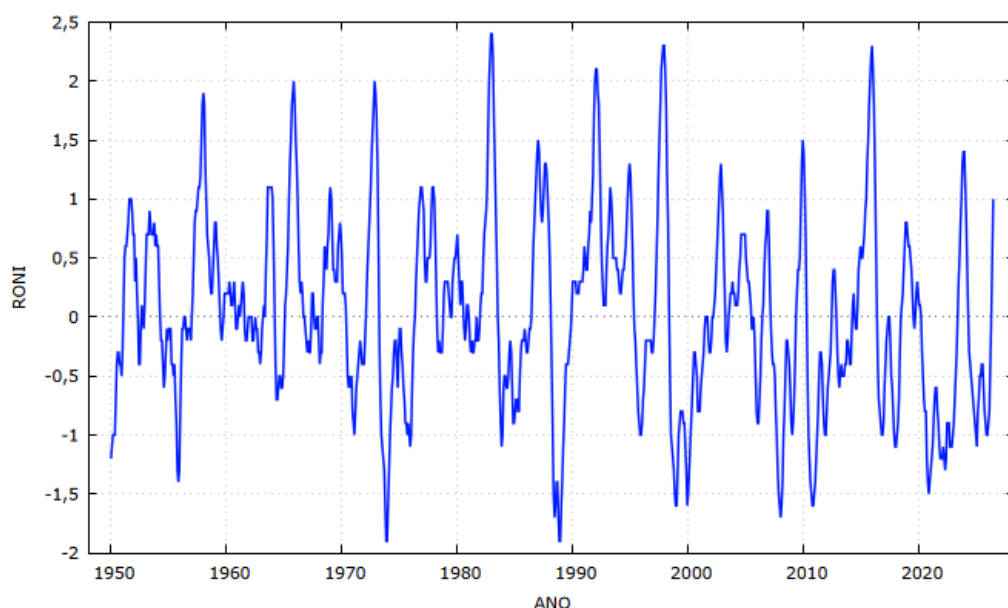
Gráfico 1 – Variação do índice oceânico Niño-RONI (1950-2026)
