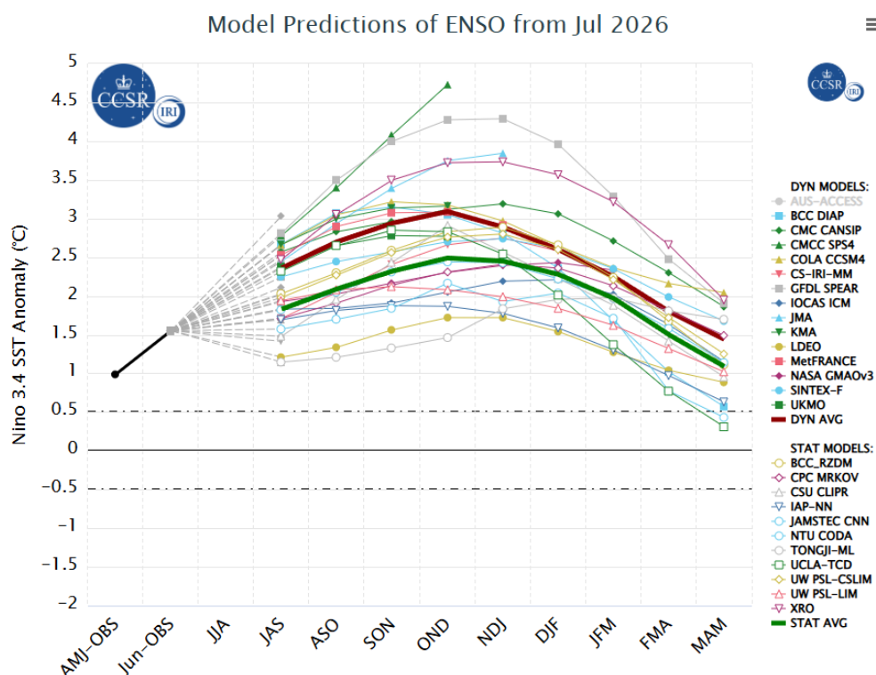
Gráfico 2 – Modelos preditivos para El-Niño
