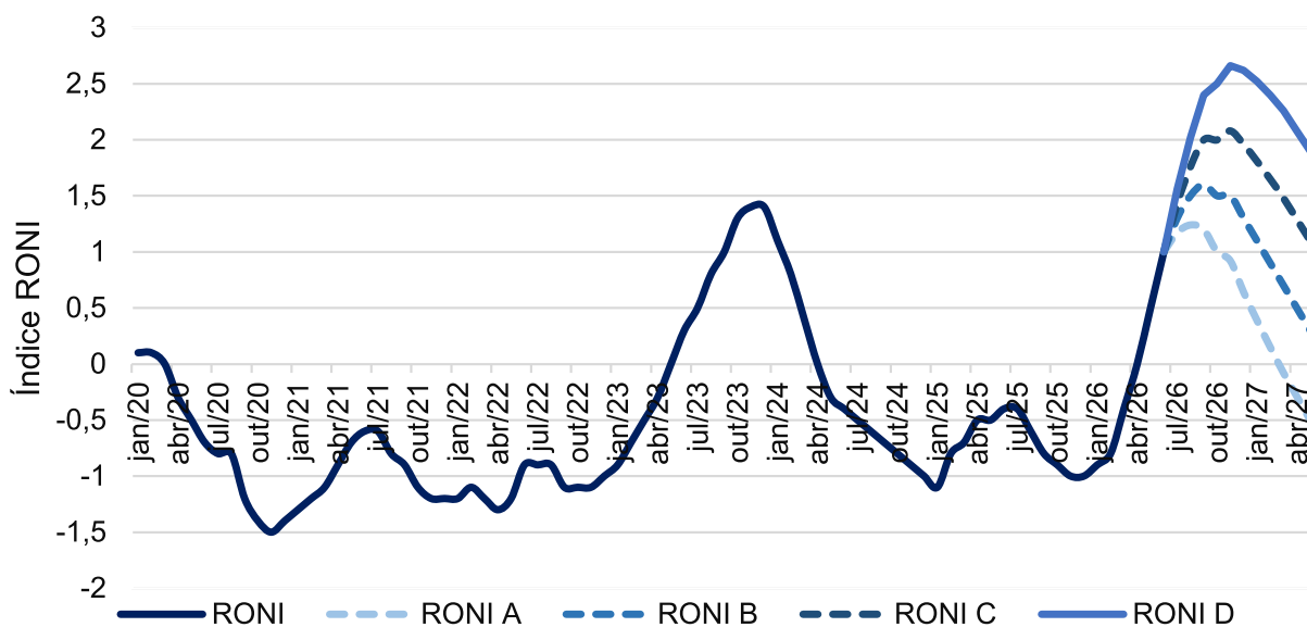
Gráfico 3 – Projeção: trajetória El-Niño
